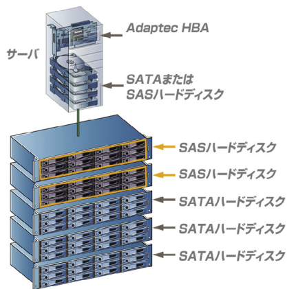
Unified Serial™アーキテクチャでのストレージ構成例
